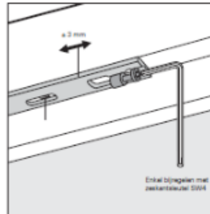
Schaar R
