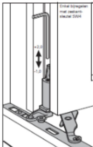
Hoekband R
