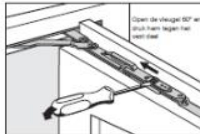
Schaar R
